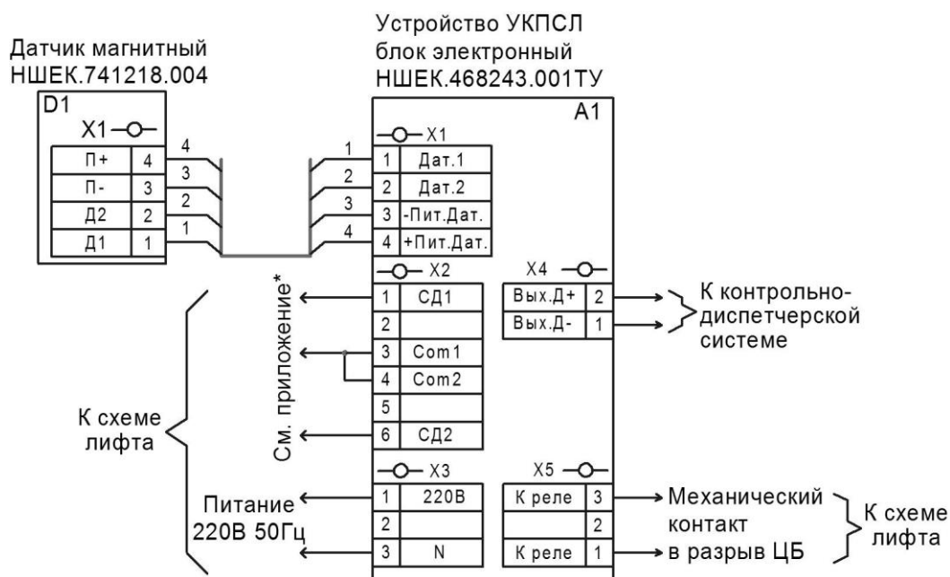
Схема подключения (для справок)
