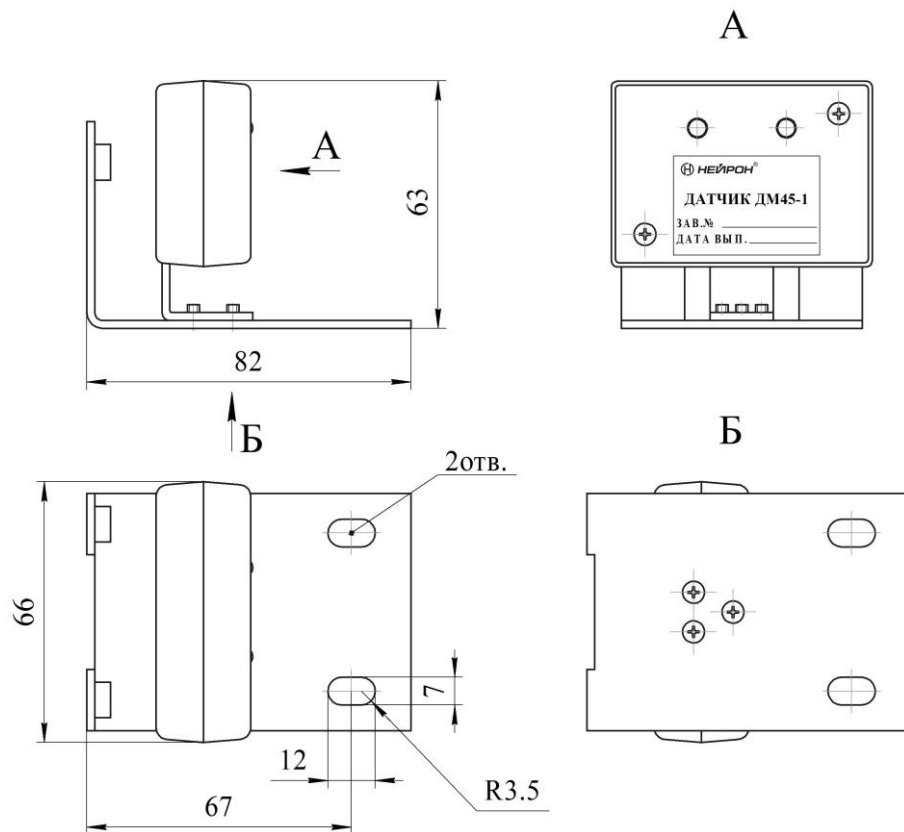
Рис. 3 Габаритный чертёж датчика магнитного ДМ45-1 НШЕК.402229.001-01
