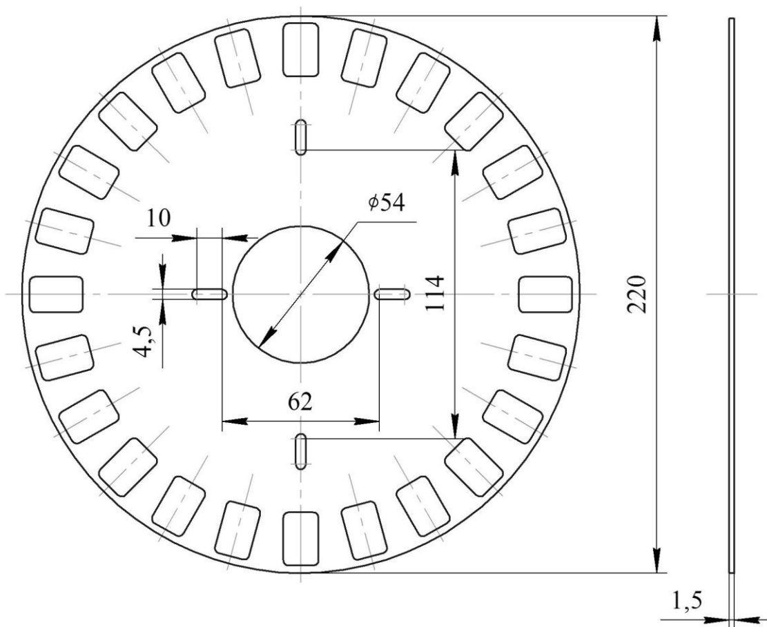
Рис. 4 Габаритный чертёж прерывателя
