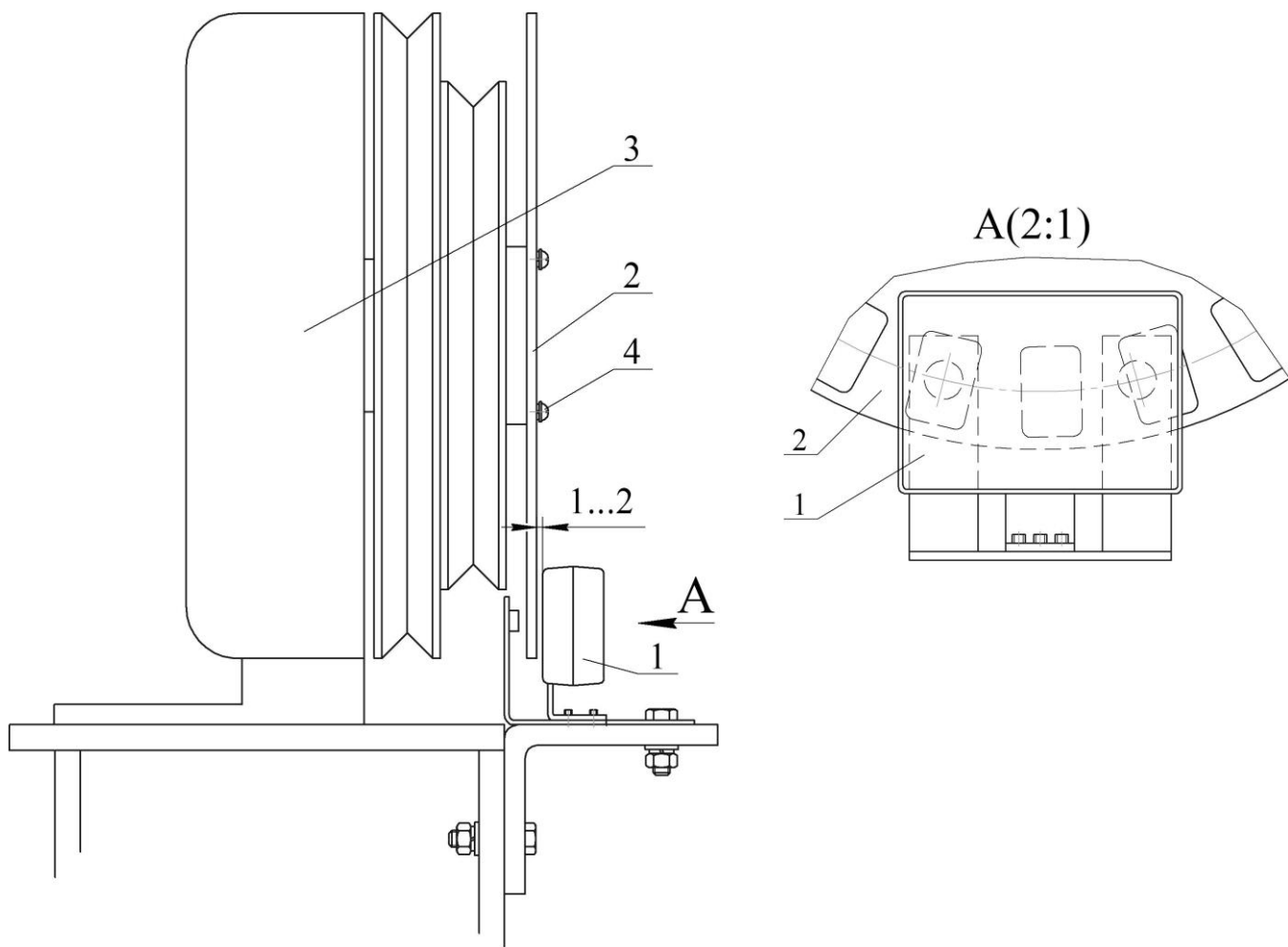
Рис. 5 Установка прерывателя и датчика магнитного ДМ45-1 НШЕК.402229.001-01 на лифты производства ЦЛЗ
